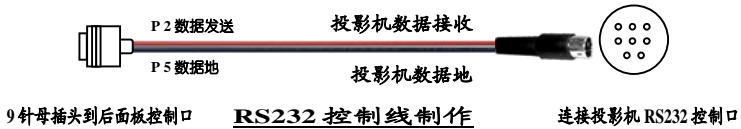
晨星 CX59、69 型投影机 RS232C 口定义
