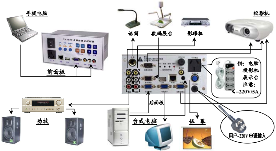
多媒体设备连接示意图
