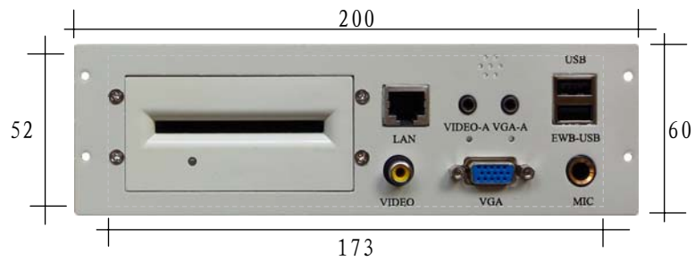
钢木讲台专用辅助面板 (带电子白板长线驱动, 2台电脑USB控制白板自动切换) 173 × 52mm 为钢木讲台安装辅助面板的开孔, 辅助面板置于钢板后方。
